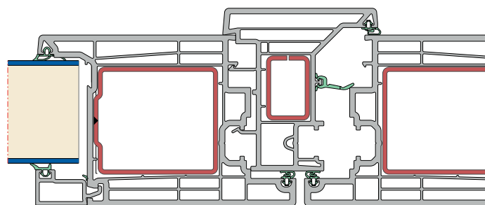
Drzwi wejściowe Elegant Infinity 76 ze słupkiem ruchomym Skala.: 1:2
