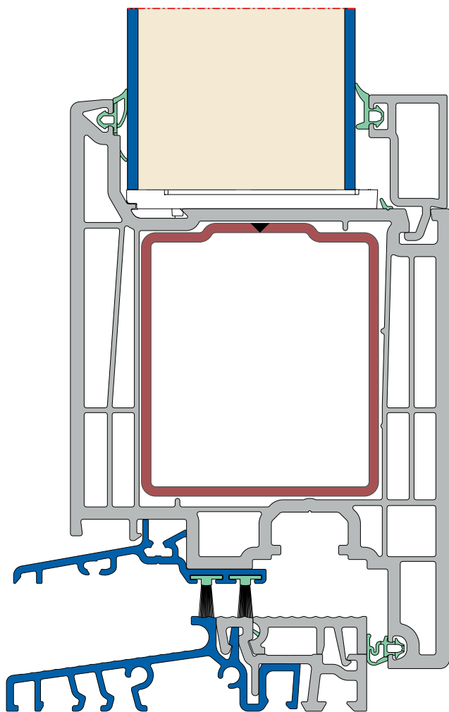
Drzwi wejściowe Elegant Infinity 76 przekrój pionowy Skala.: 1:1
