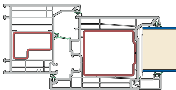
Drzwi wejściowe Elegant Infinity 76 przekrój poziomy Dormas 45 mm Skala.: 1:2
