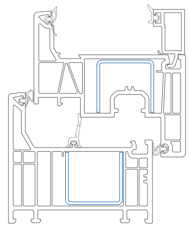
Elegant profil niezlicowany · Skala 1:2
