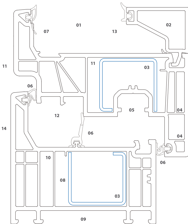
Elegant profil zlicowany Skala 1:1
