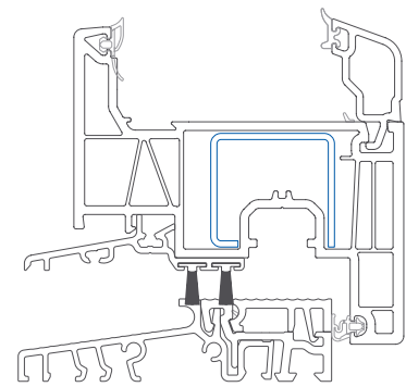
Elegant z ciepłym progiem aluminiowym i zakorągloną listwą · Skala 1:2
