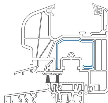
Bezbarierowy próg balkonowy / Wys. 20 mm / Rys.: 1:2
